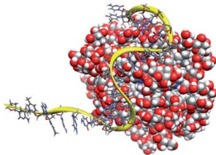
PPI dendrimer „dekorovaný“ na povrchu maltózou s navázaným oligonukleotidem ( GEM91 ). Tento komplex byl vytvořen počítačovou simulací.
