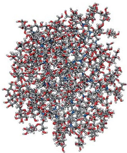
Počítačový model PPI dendrimera „dekorovaného“ na povrchu maltózou.
